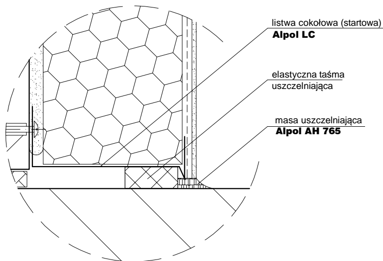
szczegół A
