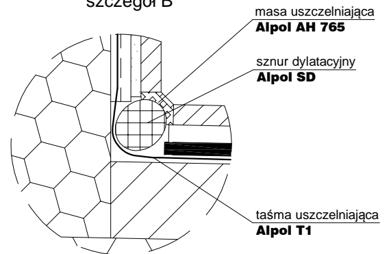
szczegół B
