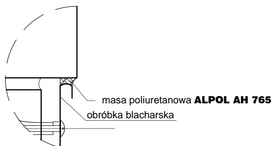
szczegół A
